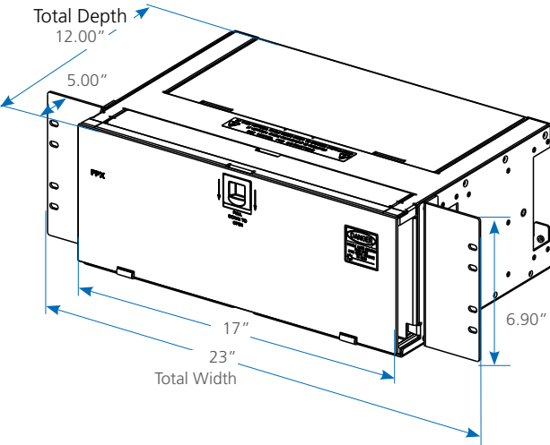
4 RU Model
